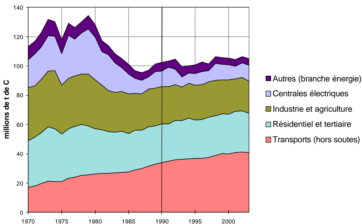
Émissions de CO 2 de la France (corrigées du climat, en millions de tonnes de carbone)
