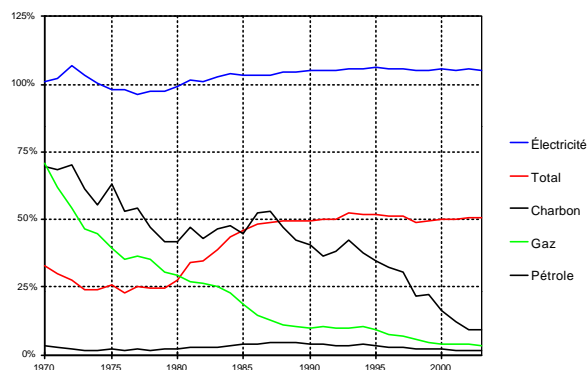
Indépendance énergétique totale et par forme d'énergie depuis 1970 (en %).
