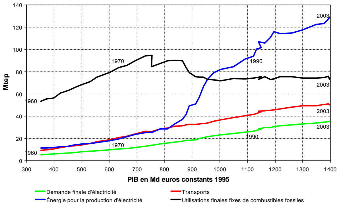
Consommation finale d'énergie par secteur, en fonction du PIB, de 1960 à 2003.
