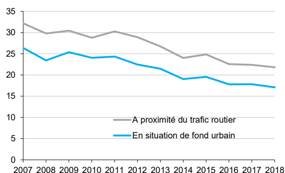
Figure D2.3-3 Évolution des concentrations annuelles en PM 10 dans l'air En µg.m -3
