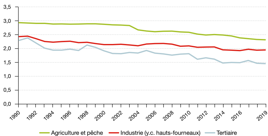
Graphique 17 : contenu carbone moyen de l'énergie par secteur En tCO 2 /tep (données corrigées des variations climatiques)
