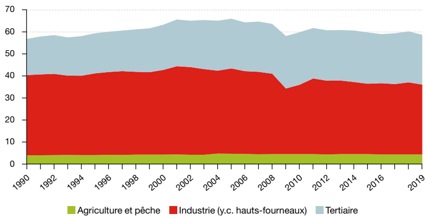
Graphique 18 : consommation d'énergie du secteur productif En Mtep (données corrigées des variations climatiques)
