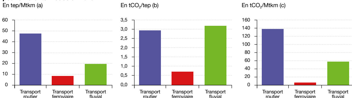
Graphique 15 : intensité énergétique (a), contenu carbone moyen de l'énergie (b) et intensité carbone (c) pour différents modes en 2019
