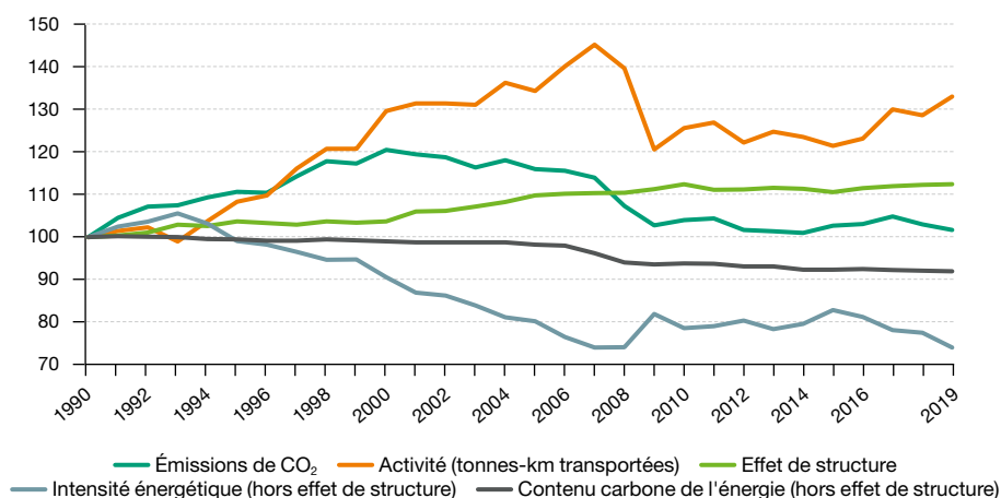
Graphique 14 : décomposition de l'évolution des émissions de CO 2 du transport de marchandises Indice base 100 en 1990
