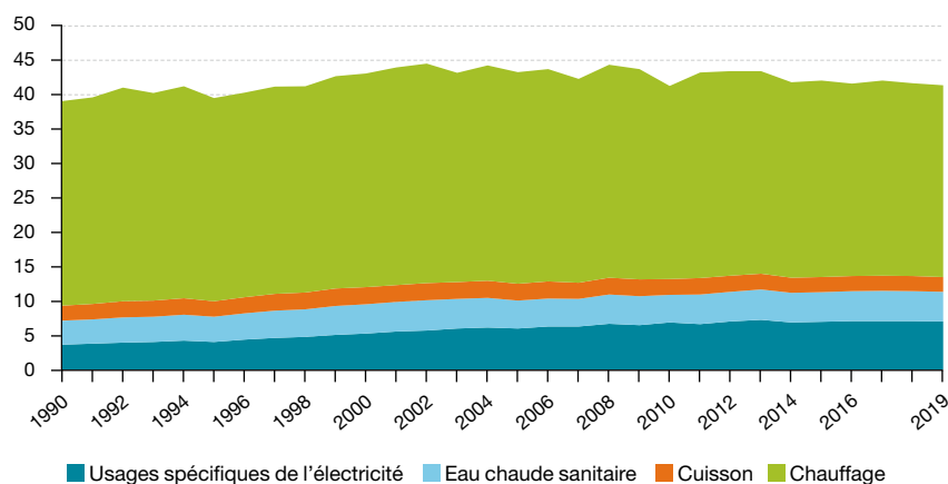
Graphique 5 : consommation d'énergie du secteur résidentiel par usage
