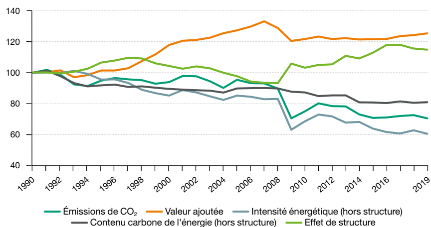
Graphique 21 : décomposition de l'évolution des émissions de CO 2 de l'industrie Indice base 100 en 1990 (données corrigées des variations climatiques)
