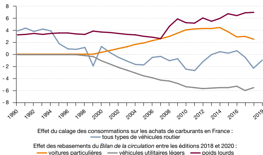
Graphique 22 : effet des principales révisions sur les émissions des transports routiers En MtCO 2
